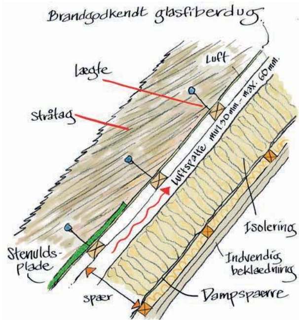
Tegning 5 Brandsikring med glasfiberdug
