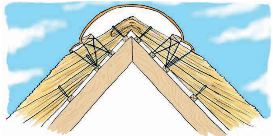
Tegning 26 Buet kobberrygning
