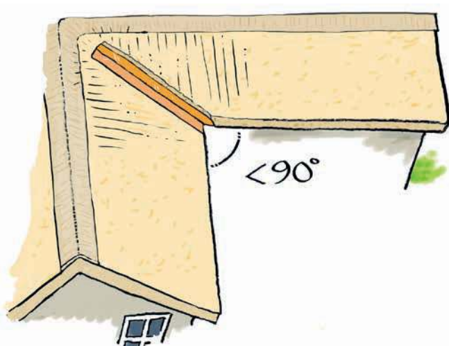
Tegning 21 Fast skotrende
