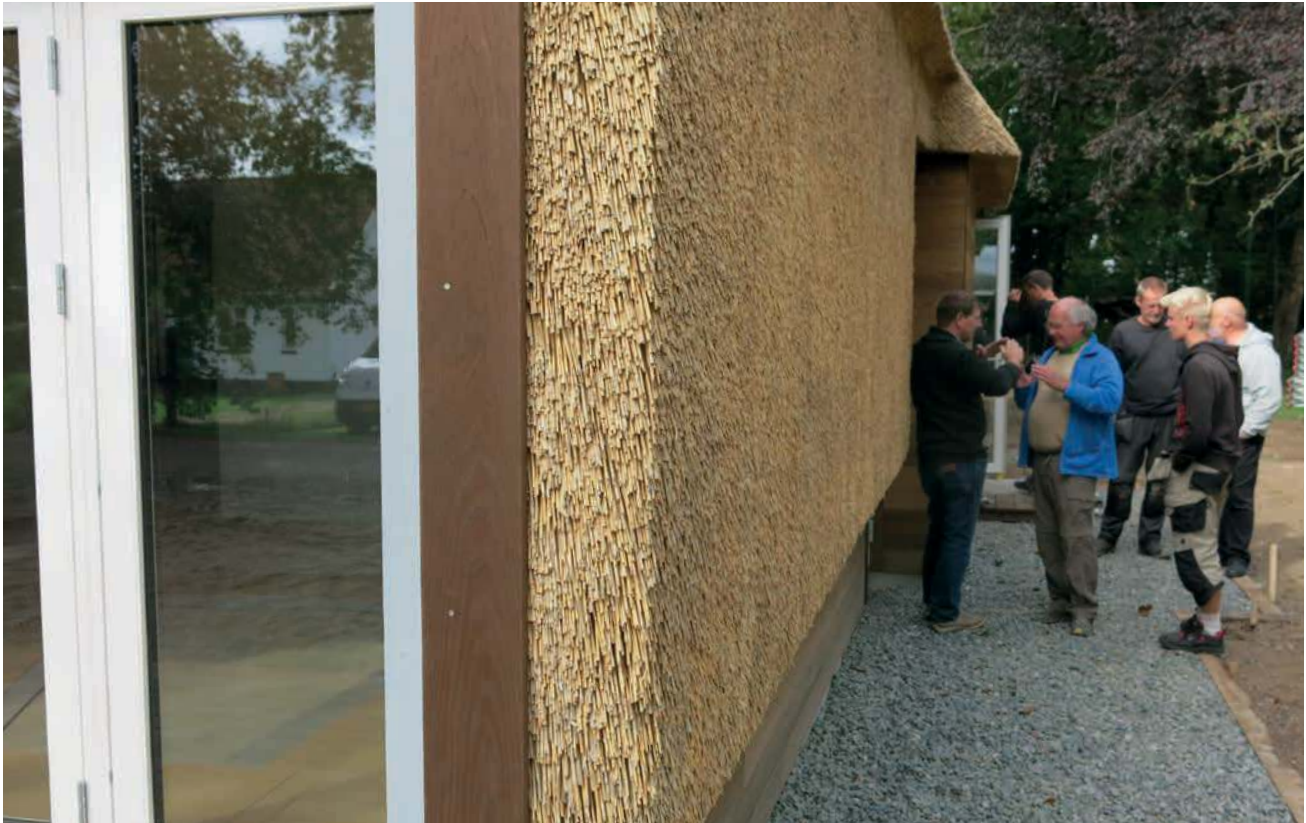
Foto 71 Lodret tækning – Det Åndbare Hus
