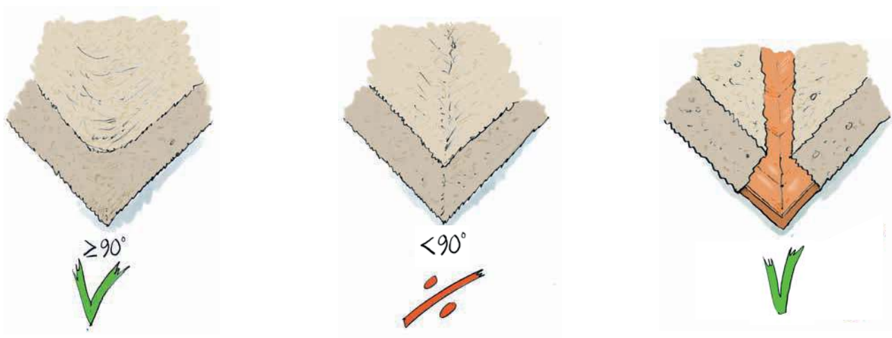
Tegning 20 Tækket skotrende / fast skotrende
